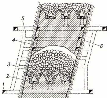
Рис. 9. Система этажного самооборудования: 1 — выработки откаточного горизонта; 2 — выработки горизонта доставки и вторичного дробления; 3 — смотровые восстающие; 4 — отрезные восстающие; 5 — выработки вентиляционного горизонта; 6 — выработки горизонтов ослабления.
